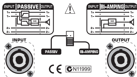
Fig. 1.1 : Panneau de connexion du subwoofer (E1800X)
