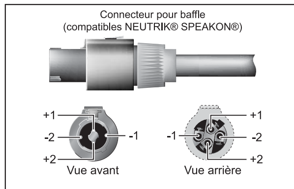
Fig. 1.2 : Connecteur Speakon®
