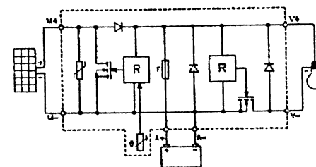
Schéma fonctionnel
