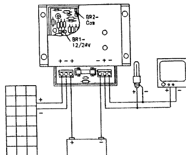
Schéma 2 : Schéma des connexions et position des cavaliers pour le réglage du développement de gaz et de tension
